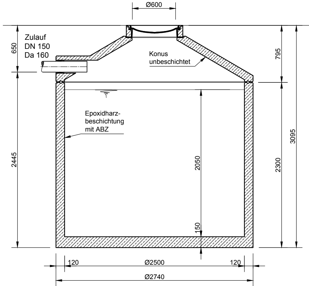
Schnitt A-A
