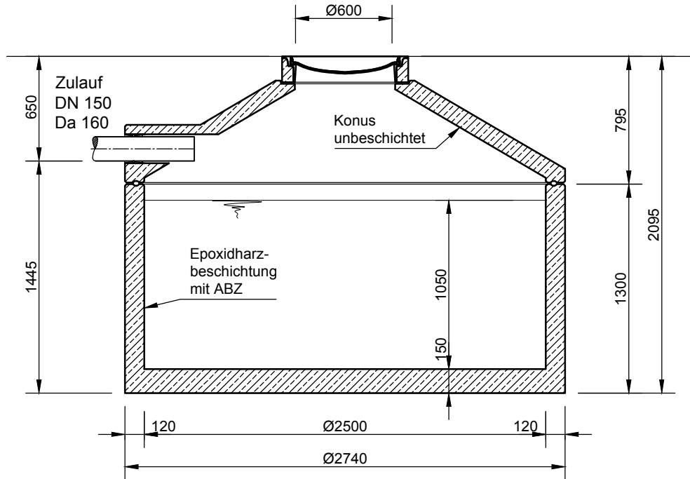
Schnitt A-A
