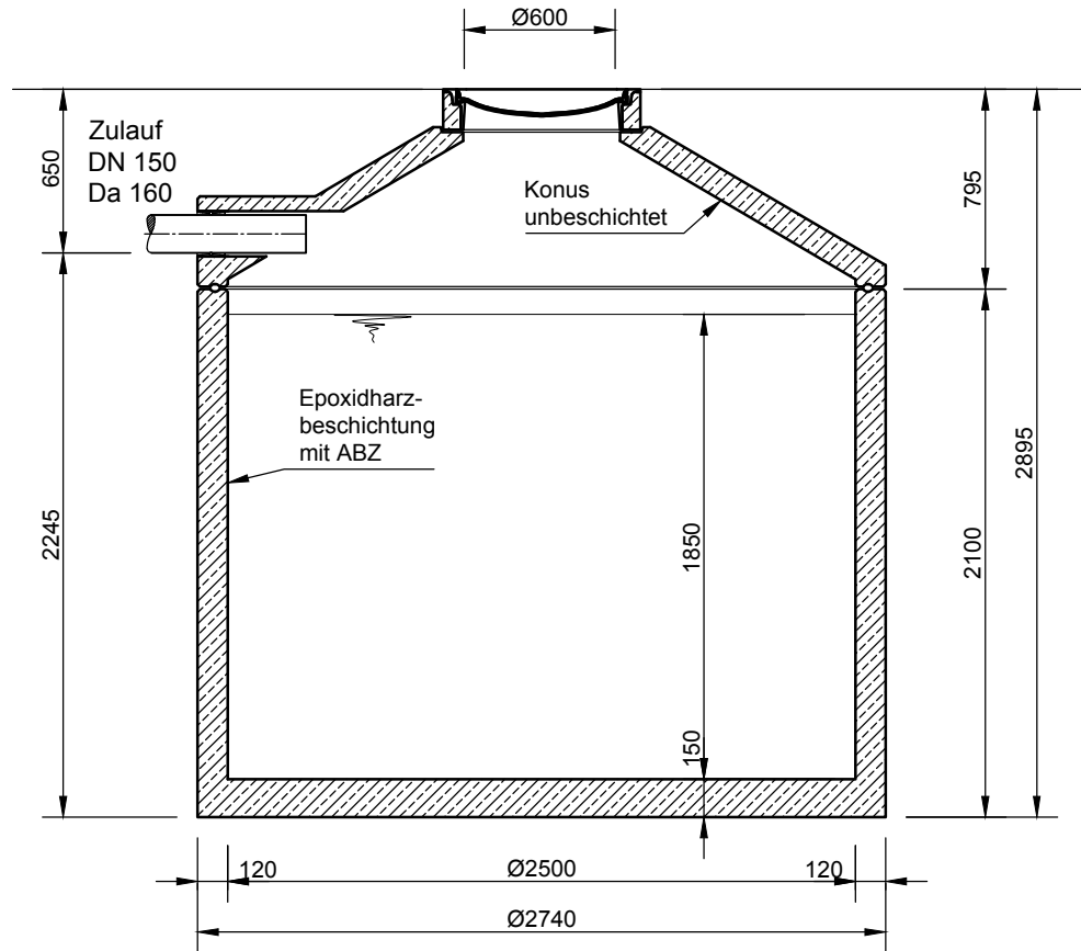
Schnitt A-A
